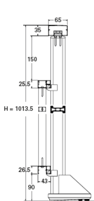
Barreaudage devant poteaux
