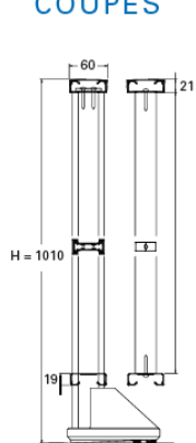
Barreaudage entre poteaux
