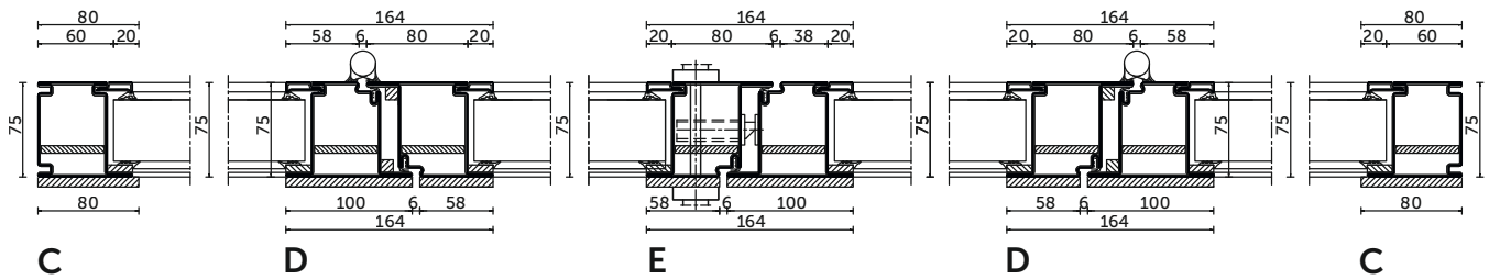
Porte à butée, à deux battants Porta a battente, a due ante
