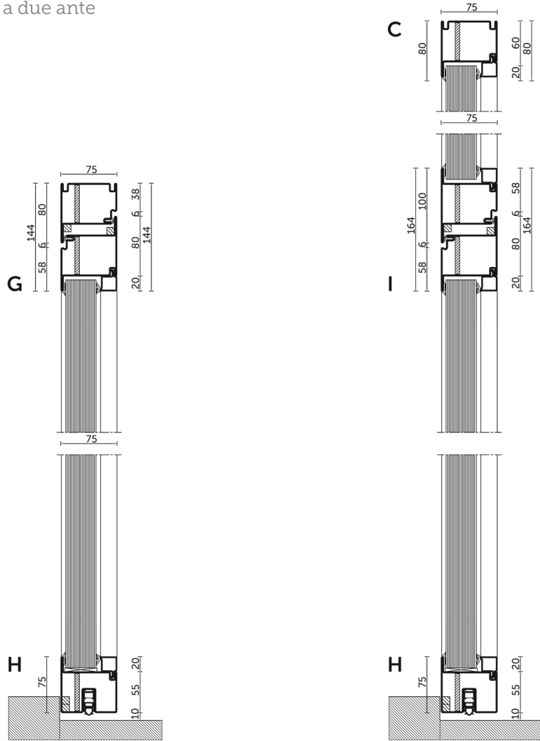
Porte à butée, s'ouvrant vers l'intérieur Porta a battente, apertura verso l'interno
