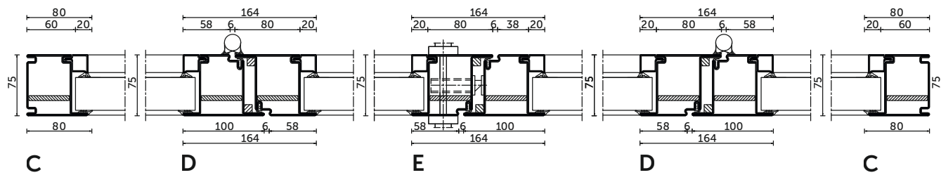
Porte à butée, à deux battants Porta a battente, a due ante
