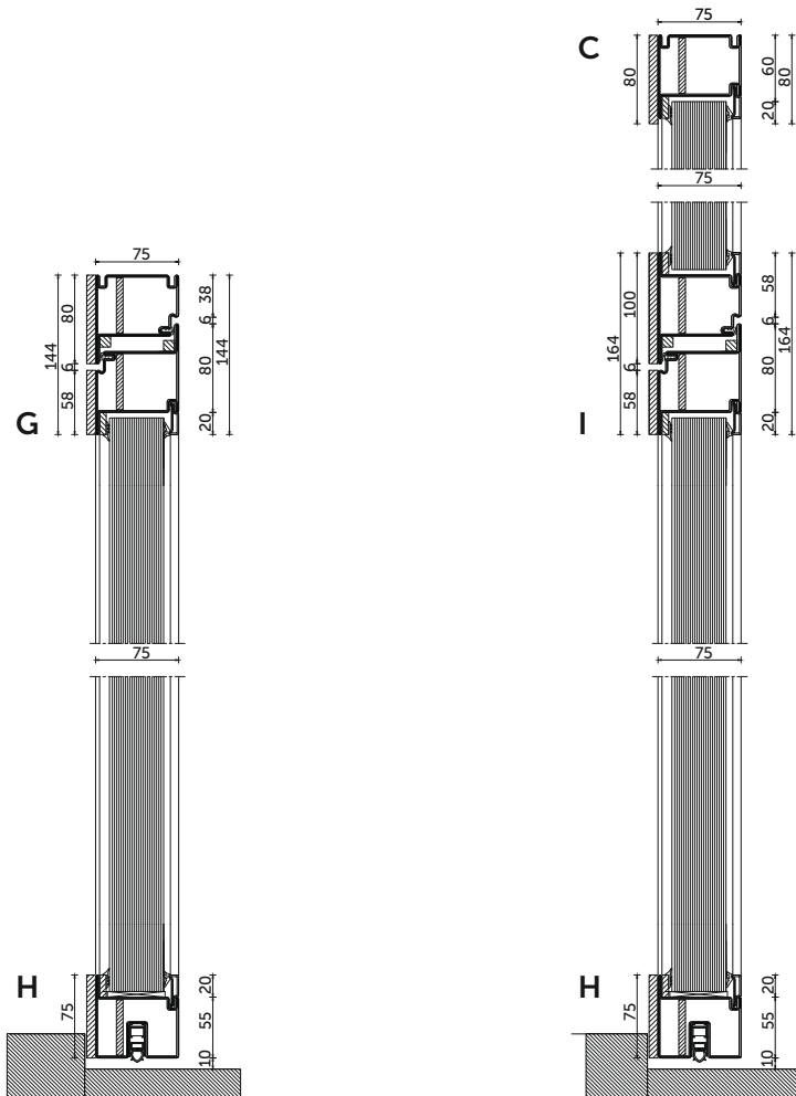
Porte à butée, à deux battants Porta a battente, a due ante
